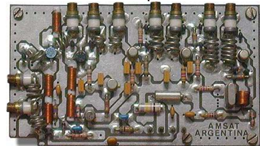
1er. equipo electrónico Argentino en el espacio, lanzado el 22 de enero de 1990, aún en órbita terrestre y funcionando
